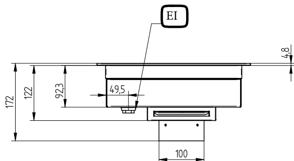
Alzado
